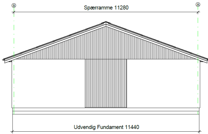
Figur 1: Gavlopstalt vest
