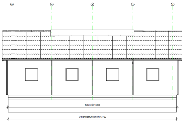
Figur 3: Sideopstalt Nord
