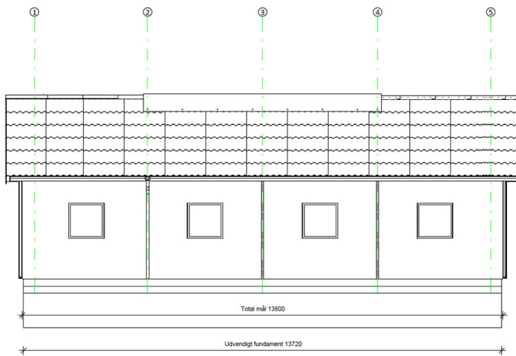
Figur 2: Sideopstalt Syd
