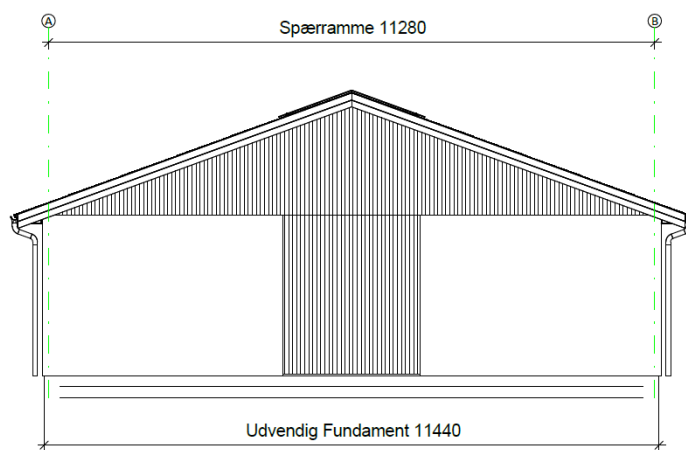
Figur 4: Gavlopstalt Øst
